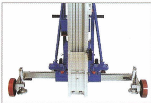
GL-850DC com as pernas frontais estendidas.
