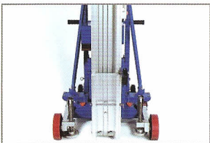
GL-850DC com as pernas frontais retraídas.
